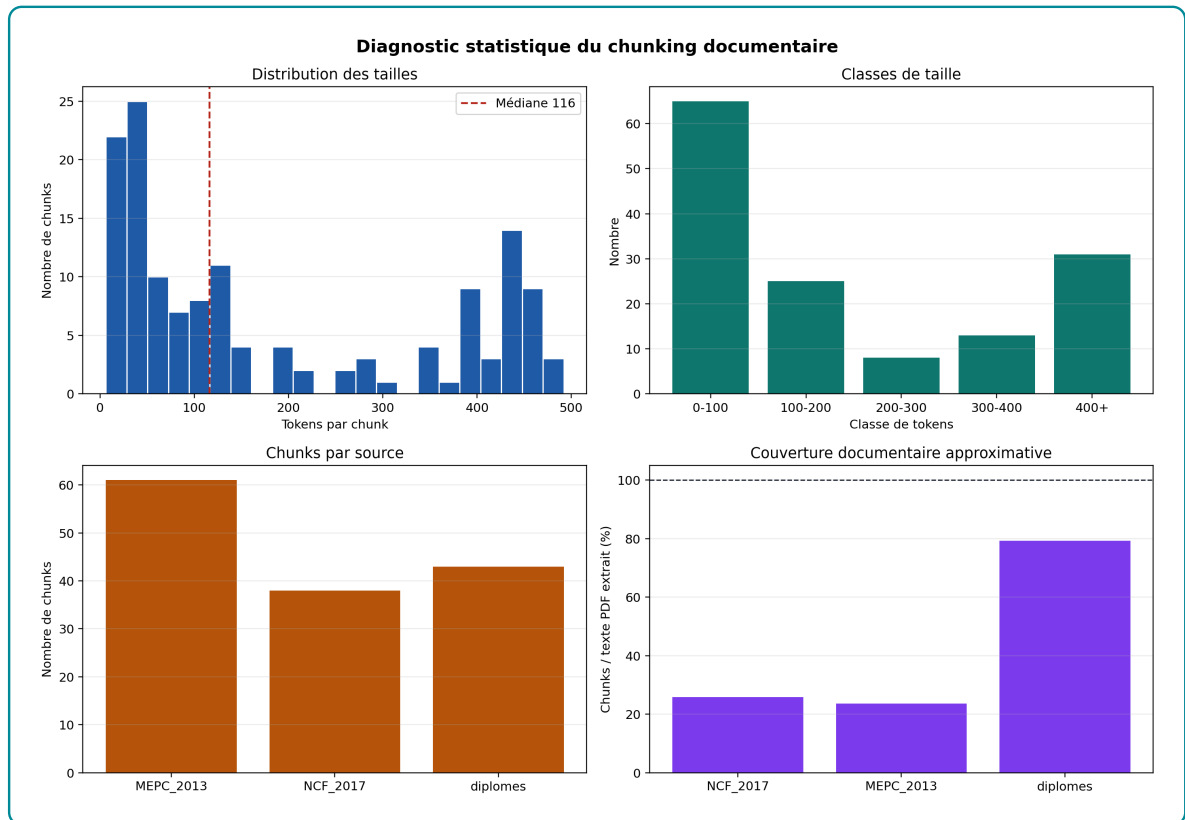
Figure 3.11 – Distribution des tailles, sources et couverture du chunking documentaire
