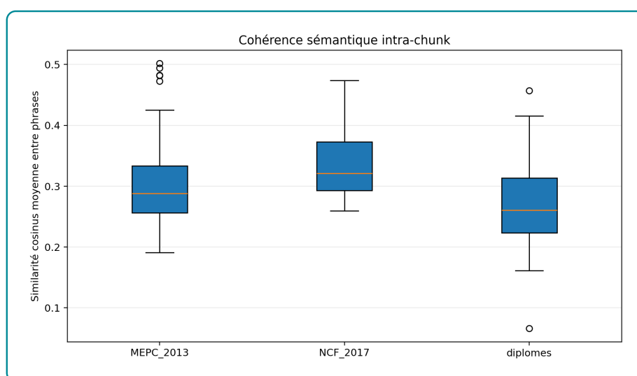
Figure 3.12 – Distribution de la cohérence sémantique intra-chunk par source
