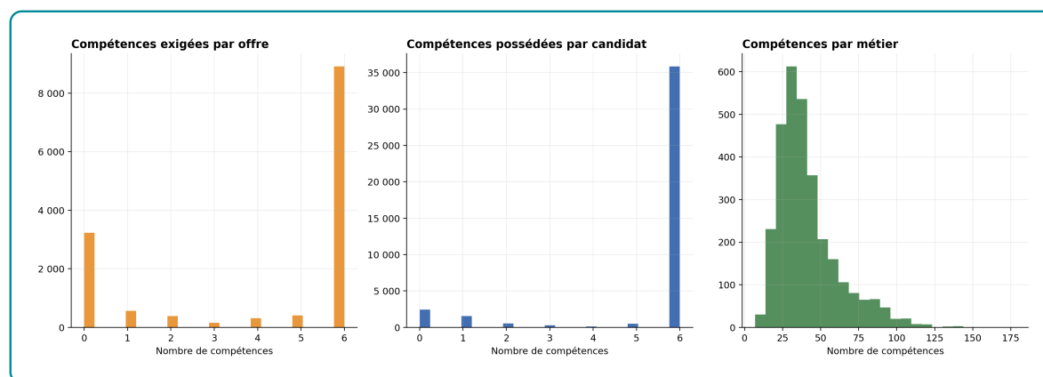
Figure 3.22 – Compétences par offre, candidat et métier dans Neo4j
