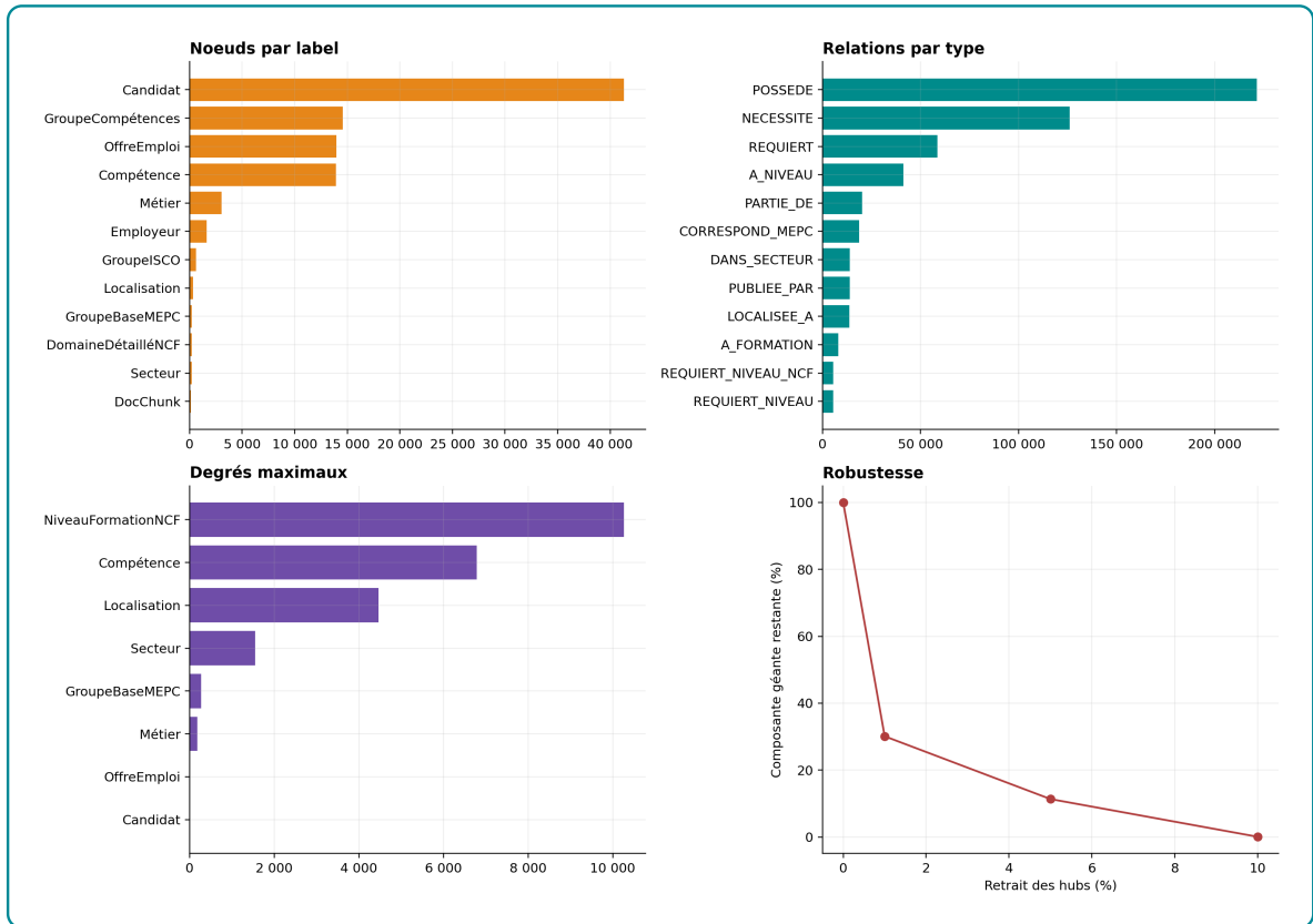
Figure 3.16 – Tableau de bord statistique du graphe Neo4j
