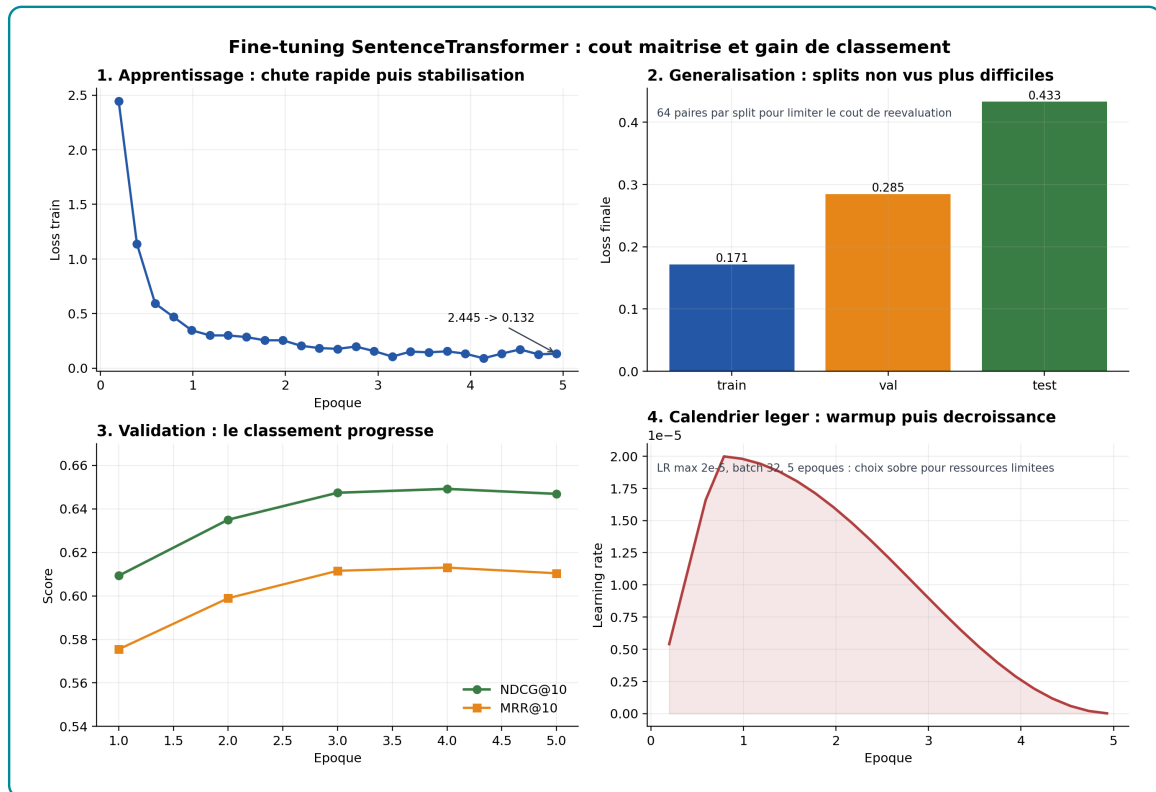
Figure 3.8 – Diagnostic du fine-tuning : perte, généralisation, métriques de validation et calendrier du learning rate
