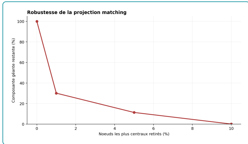
Figure 3.21 – Robustesse de la projection matching après retrait des hubs
