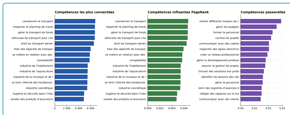
Figure 3.19 – Centralités des compétences : degré, PageRank et intermédiarité approximée
