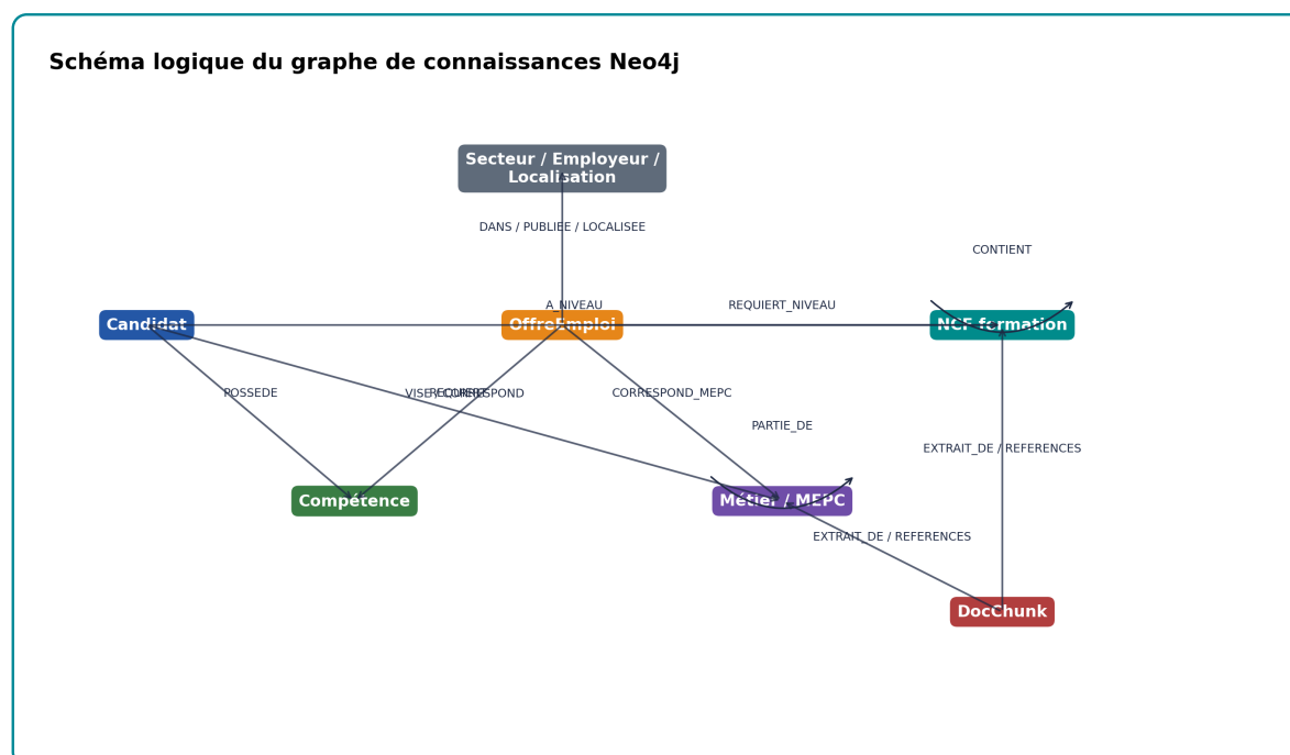
Figure 3.14 – Schéma logique du graphe de connaissances
