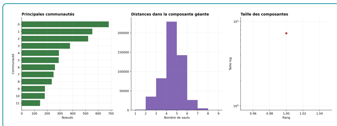
Figure 3.20 – Communautés Louvain, distances et composantes connexes
