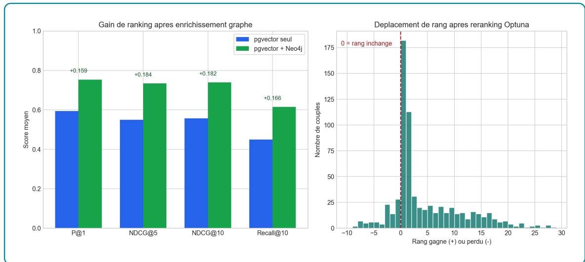
Figure 3.25 – Effet du reranking Neo4j sur les métriques et les déplacements de rang
