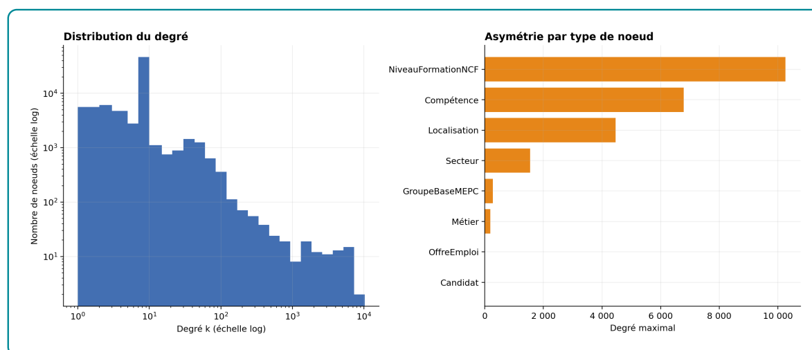
Figure 3.18 – Distribution des degrés dans la projection matching
