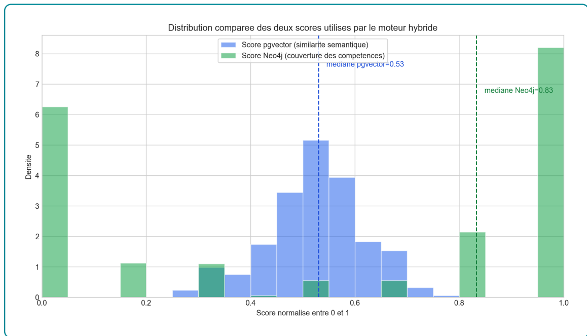
Figure 3.24 – Distribution comparée des scores pgvector et Neo4j utilisés dans le reranking
