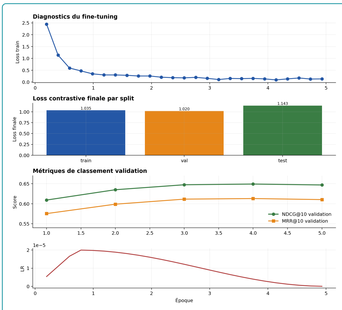
Figure 3.8 – Évolution de la perte, pertes finales par split, métriques de validation et learning rate
