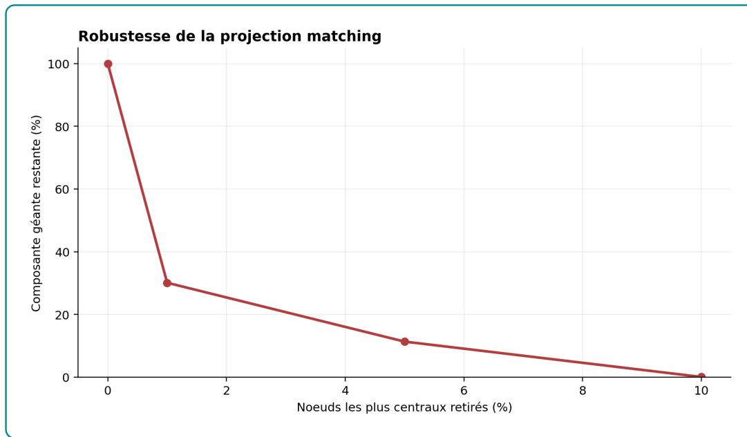
Figure A.6 – Robustesse de la projection matching après retrait des hubs
