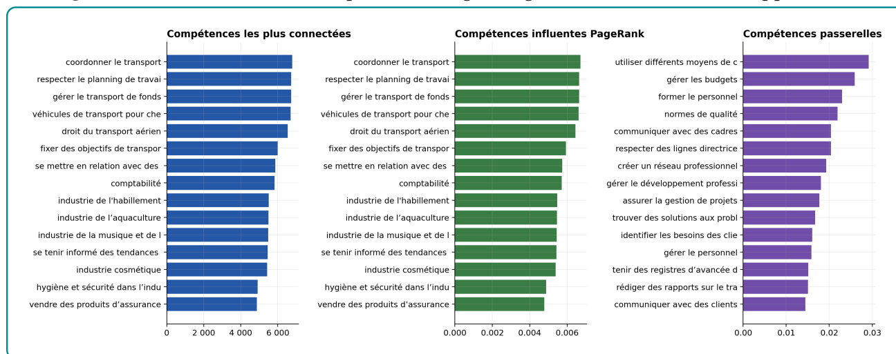
Figure A.4 – Centralités des compétences : degré, PageRank et intermédiarité approximée
