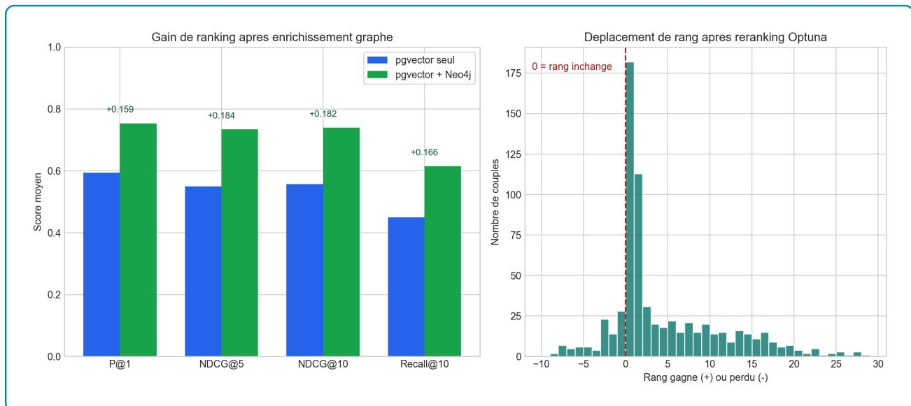
Figure 3.13 – Effet du reranking Neo4j sur les métriques et les déplacements de rang
