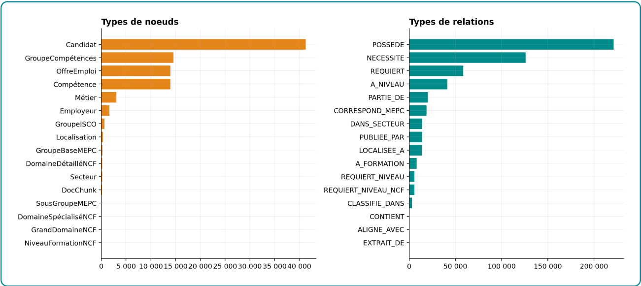
Figure A.2 – Composition du graphe par types de noeuds et relations
