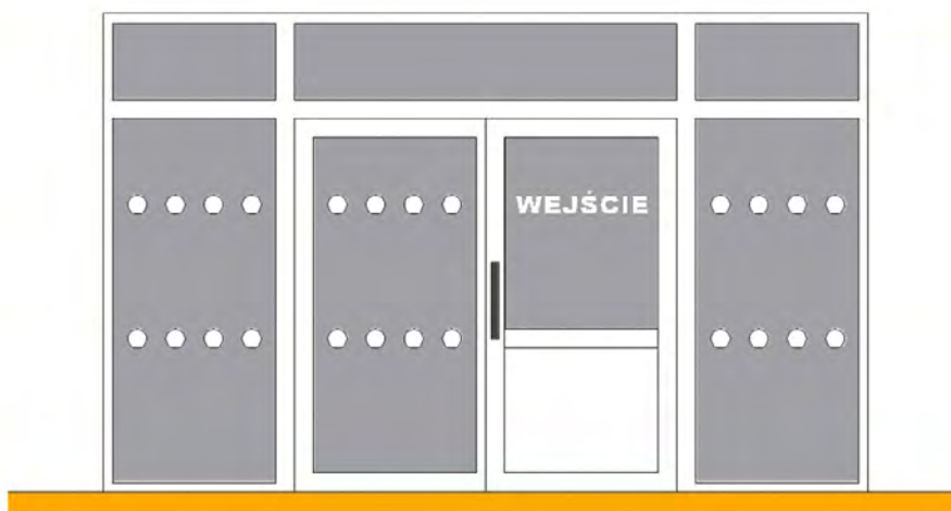
Ilustracja 9. Przykłady wyróżnienia drzwi w szklanej ścianie za pomocą koloru lub dodatkowych podziałów (rys. Katarzyna Guratowska)
