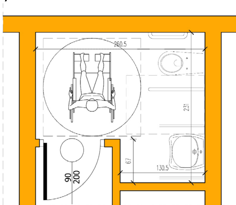
Ilustracja 17. Powierzchnia manewrowa niewystarczająca dla zapewnienia możliwości skorzystania z wszystkich elementów wyposażenia pomieszczenia (rys. Katarzyna Guratowska).
