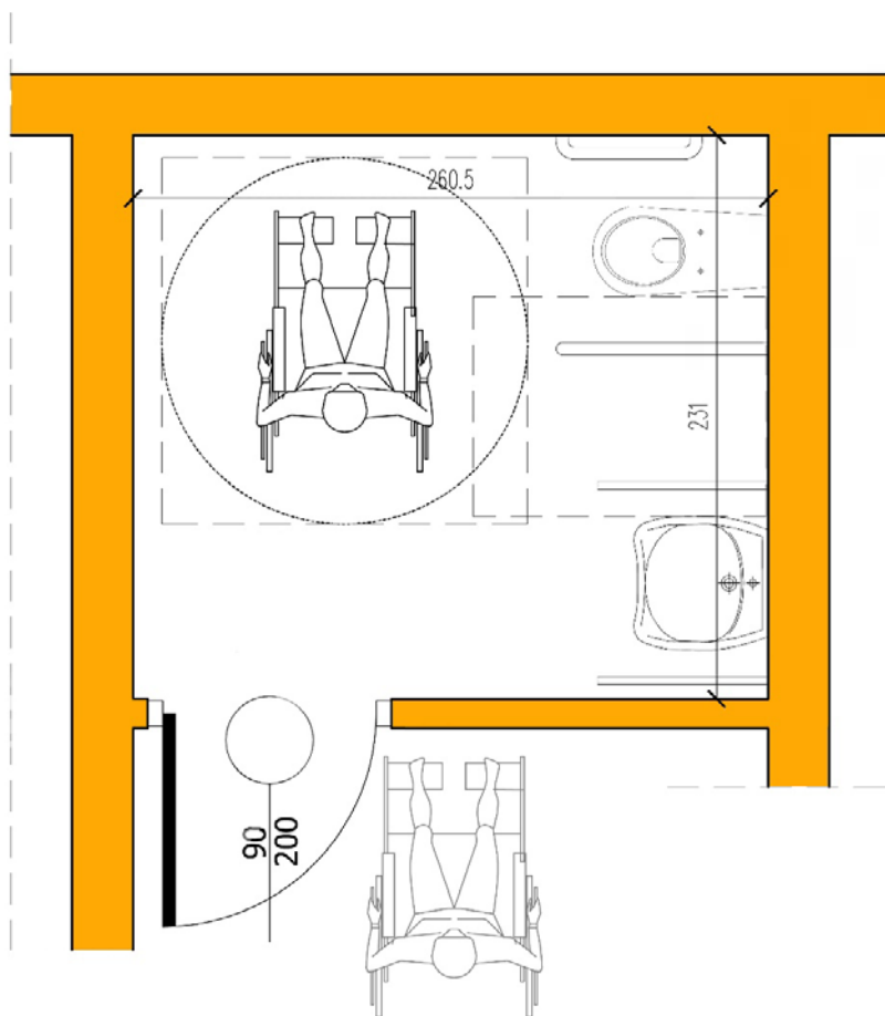
Ilustracja 18. Powierzchnia manewrowa umożliwia skorzystanie z wszystkich elementów wyposażenia pomieszczenia (rys. Katarzyna Guratowska)
