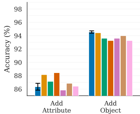
Add
