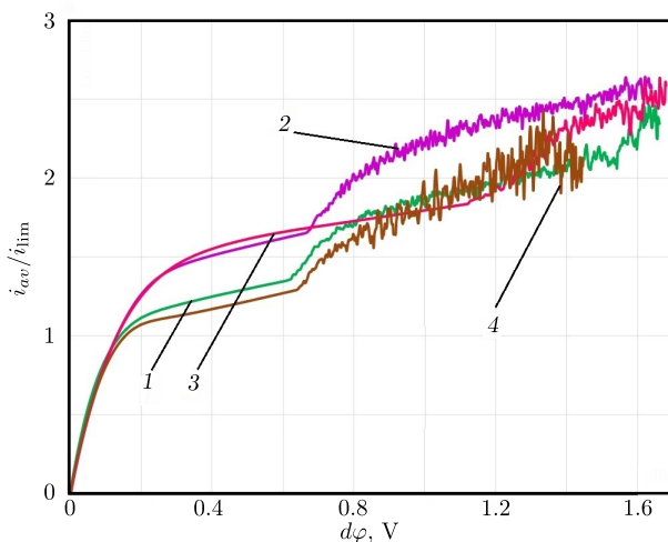
Рис. 4. (онлайн в цвете) ВАХ, соответствующие каналам обессоливания электро-диализного аппарата с раствором NaCl без спейсеров (1) и с включением только спейсеров круглой формы в центре канала (2) и при их смещении влево (3) и вправо (4) от центра, представленных на рис. 3
