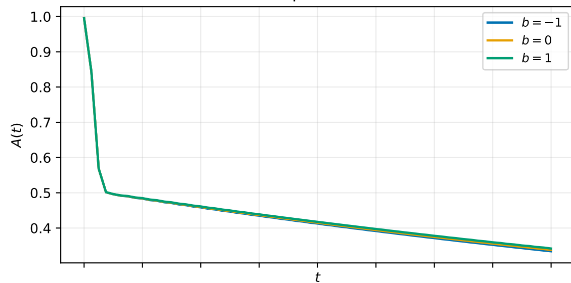
a = 2 : amplitude máxima
