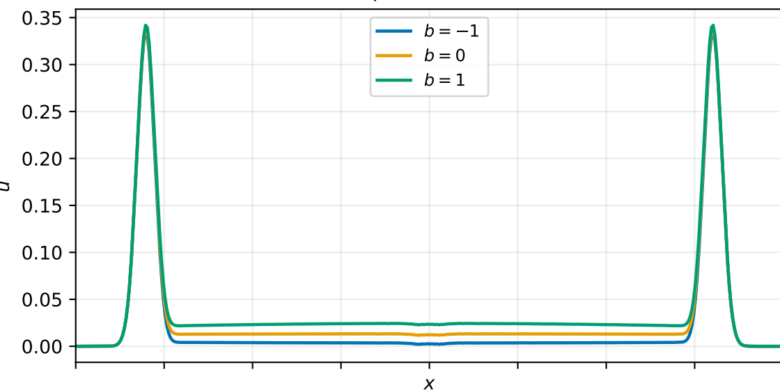
a = 2 : perfis em t = 0.8
