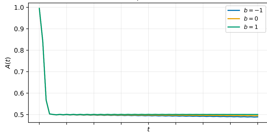
a = 1 : amplitude máxima
