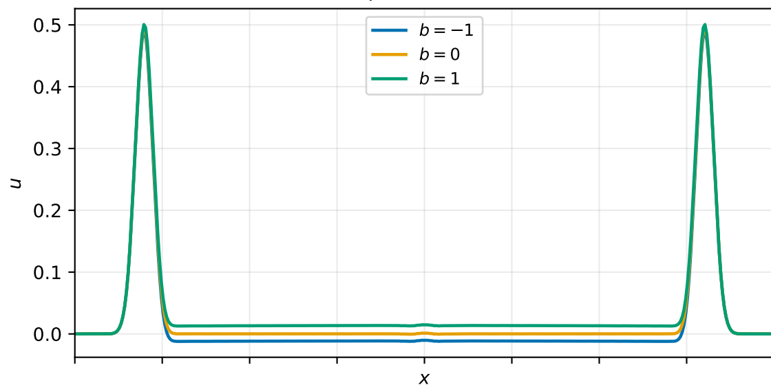
a = 1 : perfis em t = 0.8
