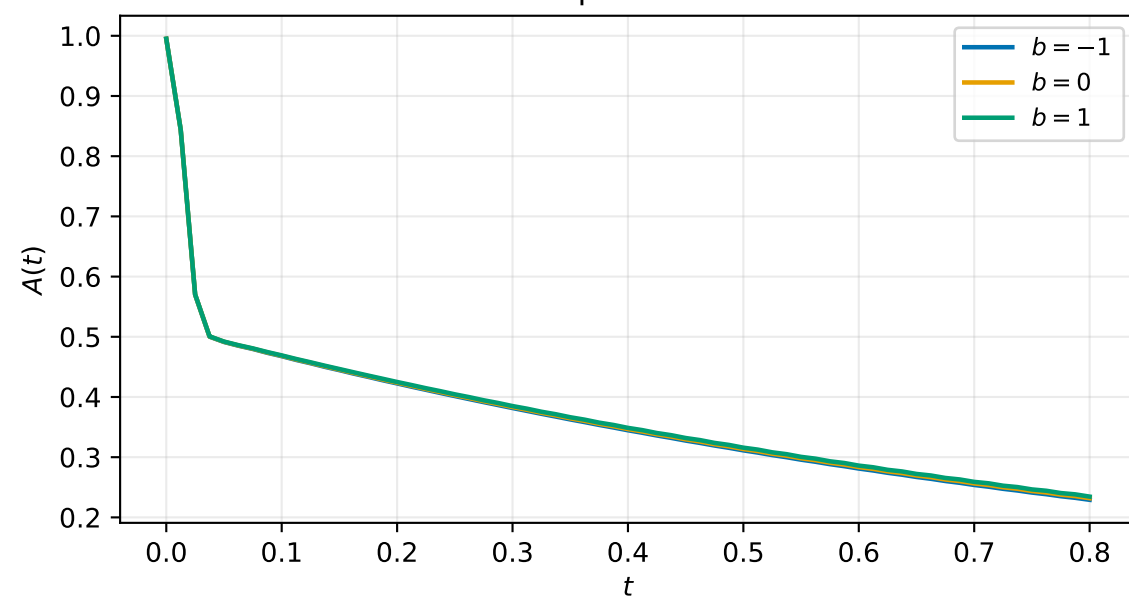
a = 2 : amplitude máxima
