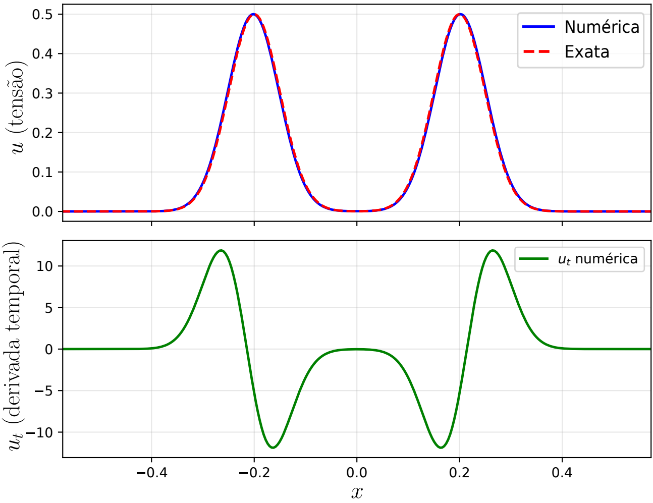
Malha (N = 1024) — t = 0.10
