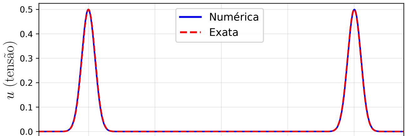
Malha (N = 1024) — t = 0.50
