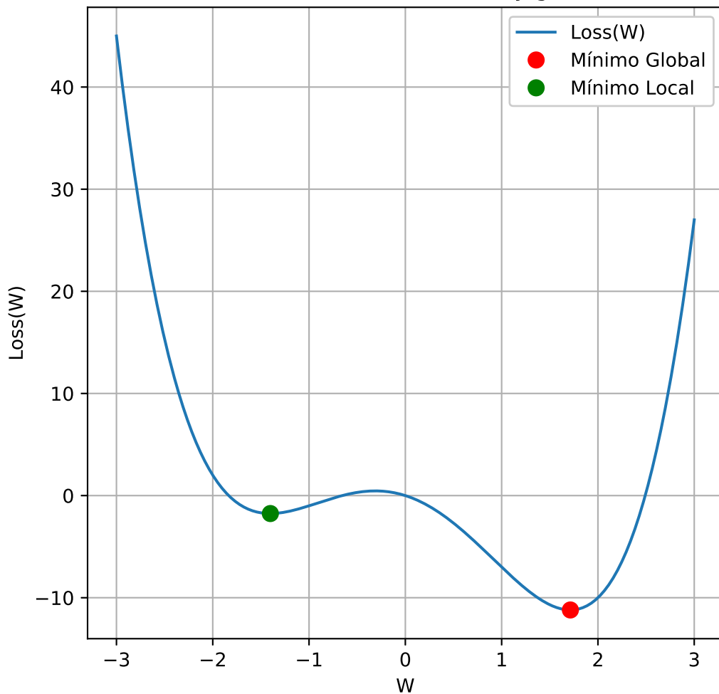
Función con mínimos local y global
