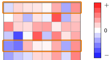
Input X
