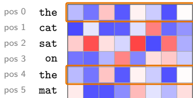
Token embedding
