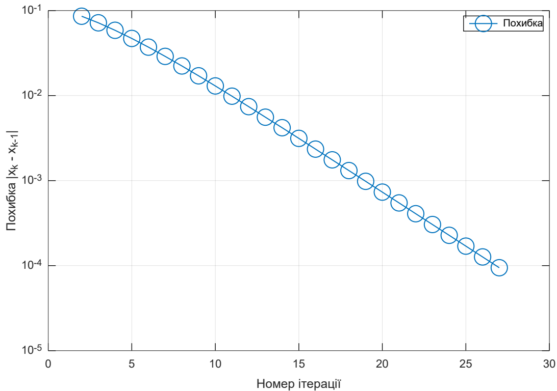
Зміна похибки від номера ітерації (метод хорд)
