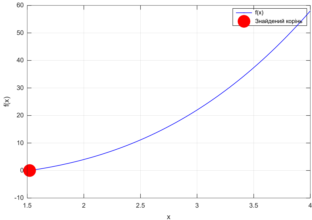
Графік функції та знайдений корінь (метод хорд)
