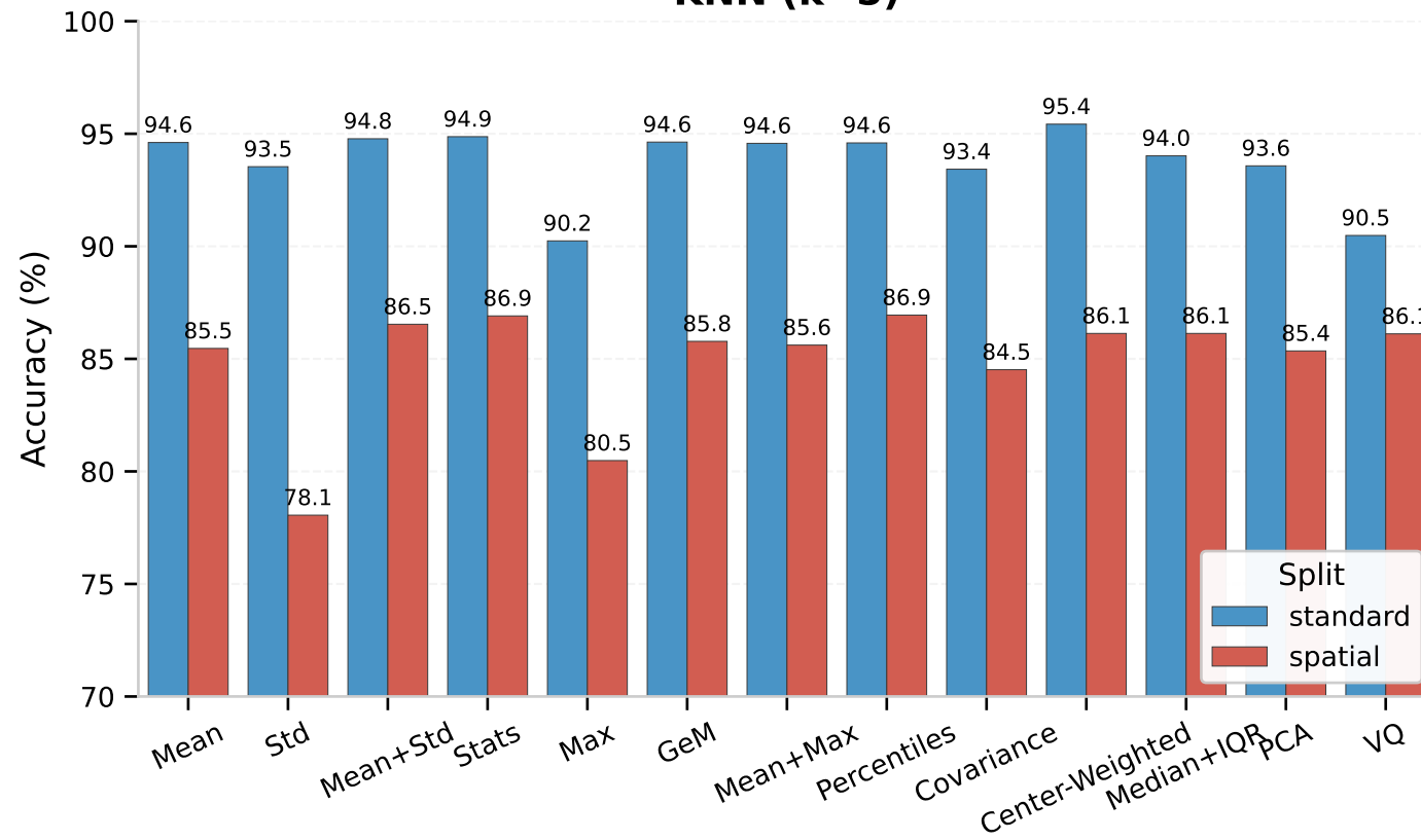
KNN (k=5)
