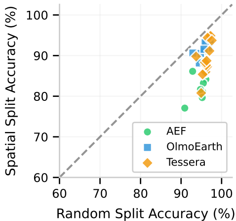
Linear Probe
