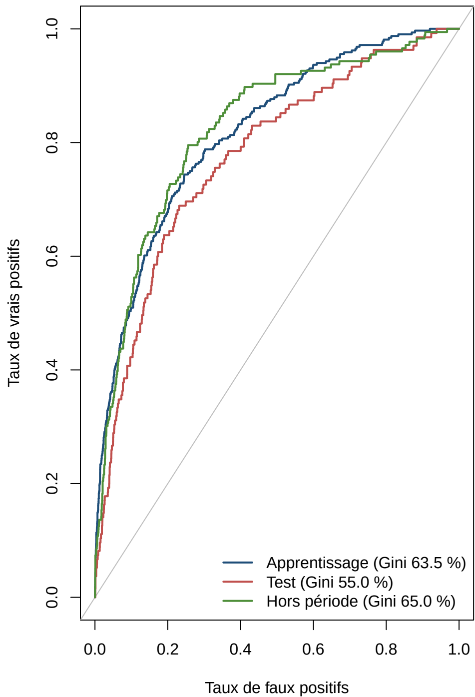
Courbes ROC
