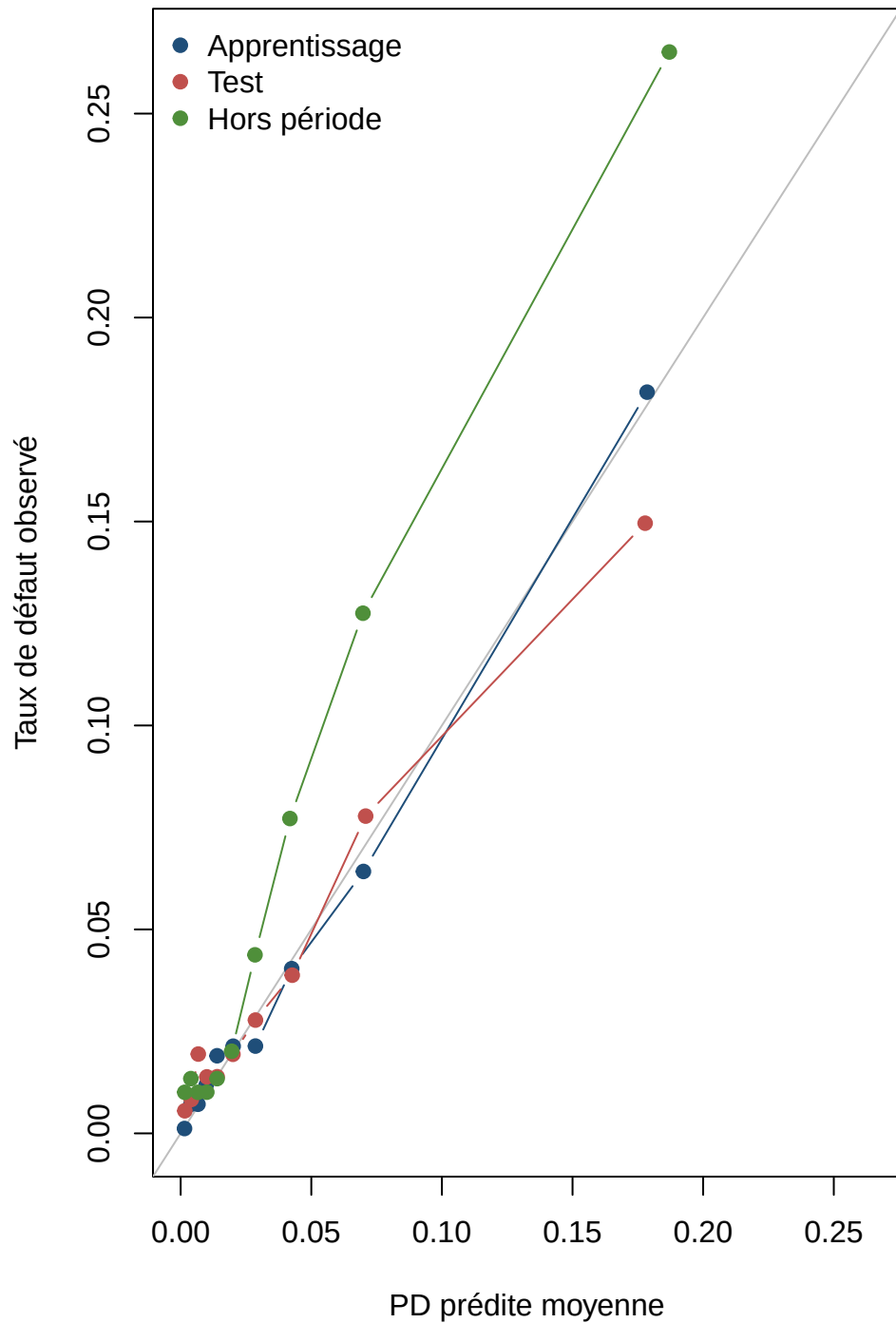
Calibration par déciles
