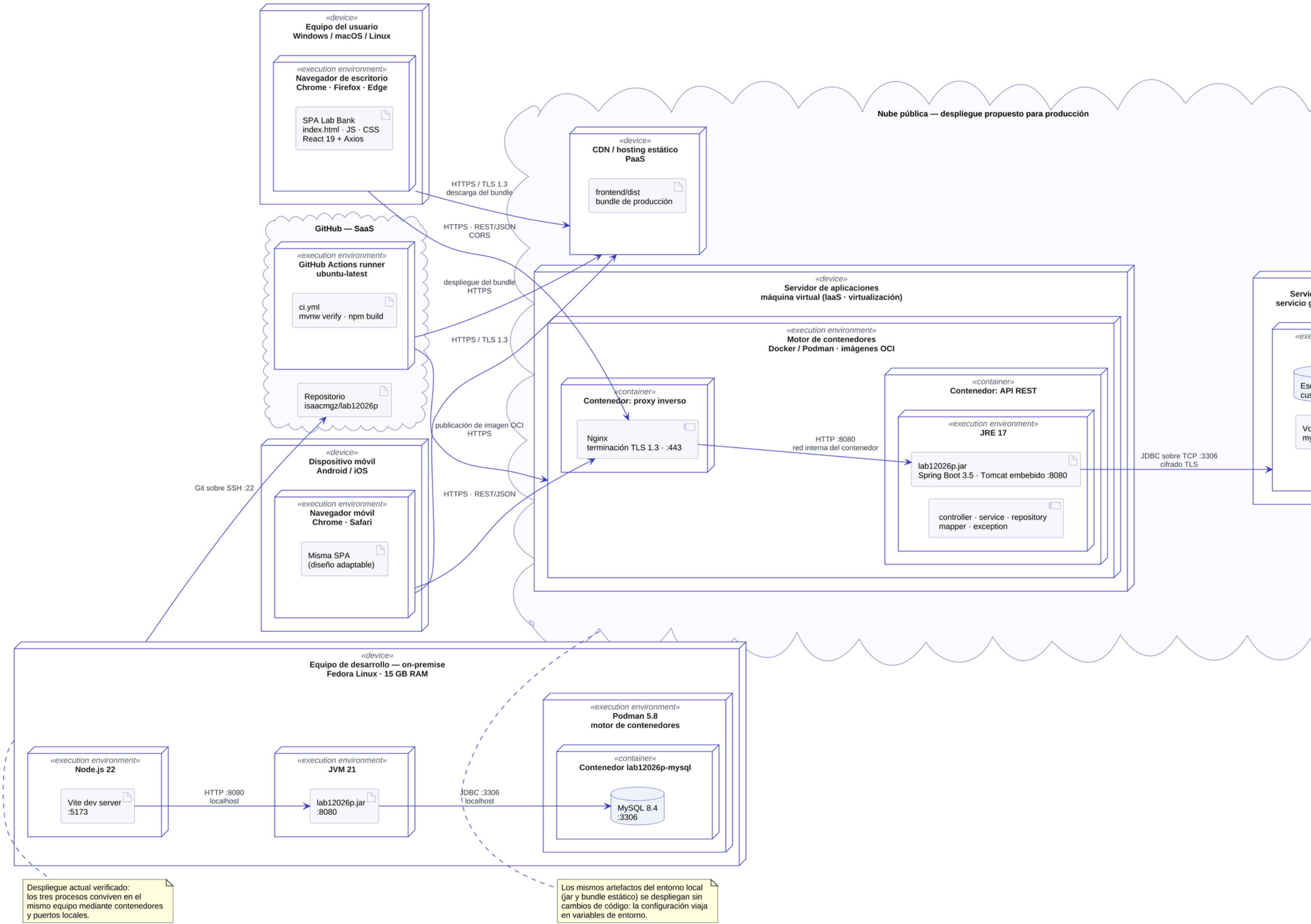
Diagrama de despliegue — Sistema bancario "Lab Bank"
