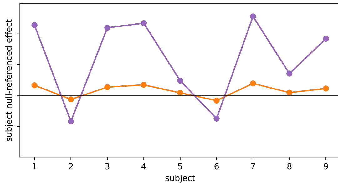
1test · LE
