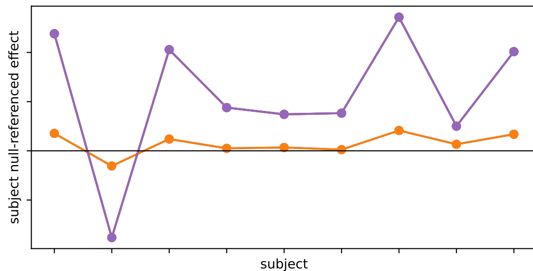
1test · LE
