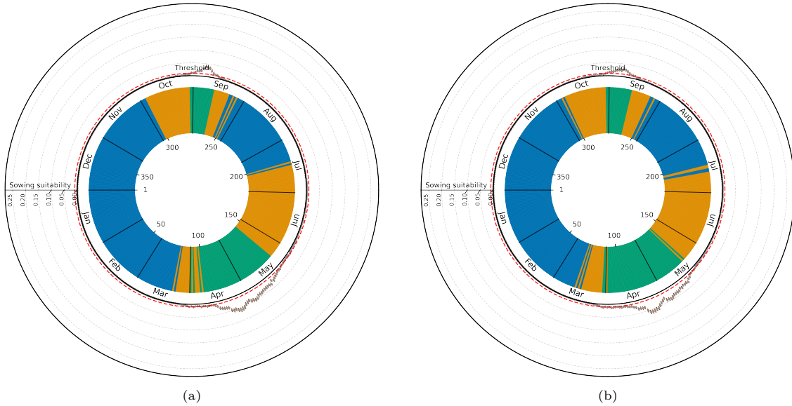
Figura 8: Calendario de los periodos de siembra identificados para Sajonia mediante las distancias Euclidiana y Manhattan. Las figuras 8a y 8b muestran los periodos resultantes para cada distancia, respectivamente.
