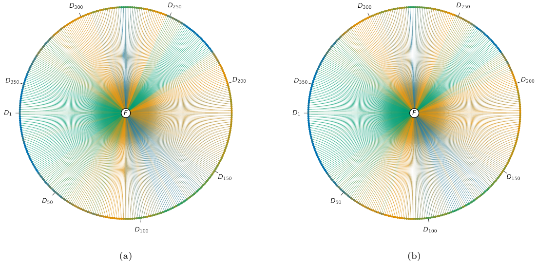
Figura 5: Aptitud diaria para la siembra en Sajonia, expresada como la probabilidad de transición \lambda_k , k \in \{1, 2, \dots, 365\} , calculada mediante las distancias Euclidiana y Manhattan. La figura 5a muestra los valores de \lambda_k calculados mediante la distancia Euclidiana, mientras que la figura 5b muestra los valores correspondientes calculados mediante la distancia Manhattan. La progresión del año se expresa en sentido contrario a las manecillas del reloj; en el exterior de la gráfica anular se indican los meses, mientras que en su interior se indican los días del año.
