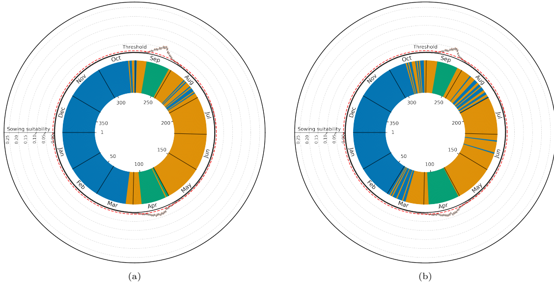
Figura 9: Calendario de los periodos de siembra identificados para Baviera mediante las distancias Euclidiana y Manhattan. Las figuras 9a y 9b muestran los periodos resultantes para cada distancia, respectivamente.
