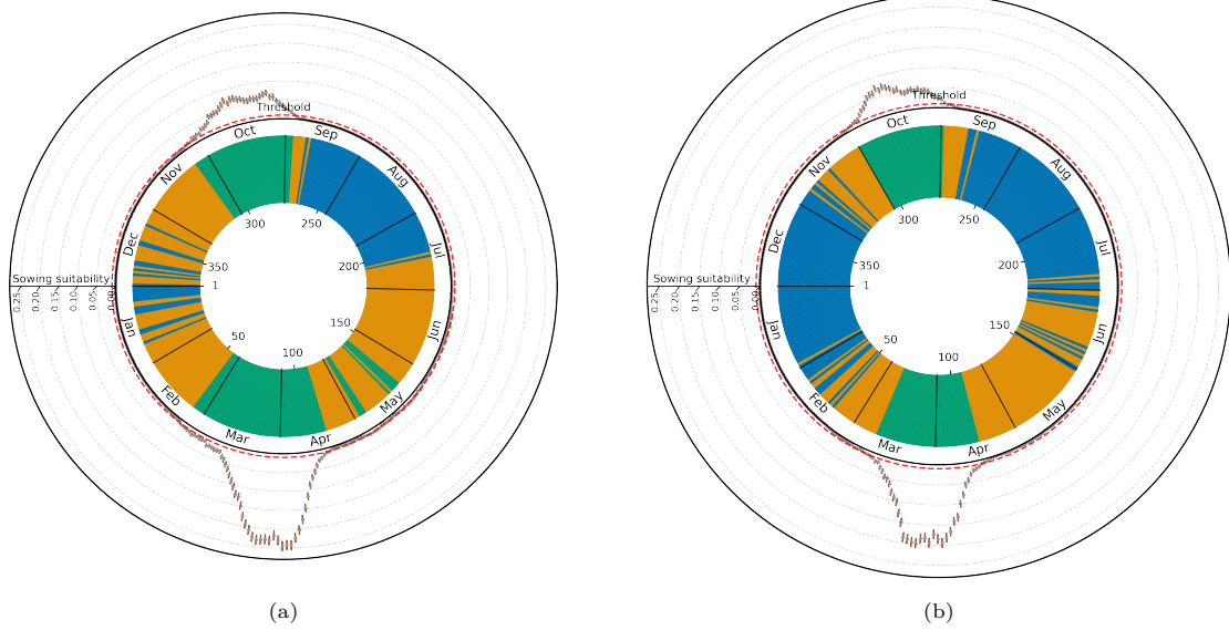
Figura 7: Calendario de los periodos de siembra identificados para Brandenburg mediante las distancias Euclidiana y Manhattan. Las figuras 7a y 7b muestran los periodos resultantes para cada distancia, respectivamente.
