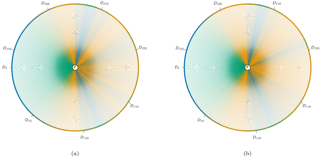
Figura 6: Aptitud diaria para la siembra en Baviera, expresada como la probabilidad de transición \lambda_k , k \in \{1, 2, \dots, 365\} , calculada mediante las distancias Euclidiana y Manhattan. La figura 6a muestra los valores de \lambda_k calculados mediante la distancia Euclidiana, mientras que la figura 6b muestra los valores correspondientes calculados mediante la distancia Manhattan. La progresión del año se expresa en sentido contrario a las manecillas del reloj; en el exterior de la gráfica anular se indican los meses, mientras que en su interior se indican los días del año.
