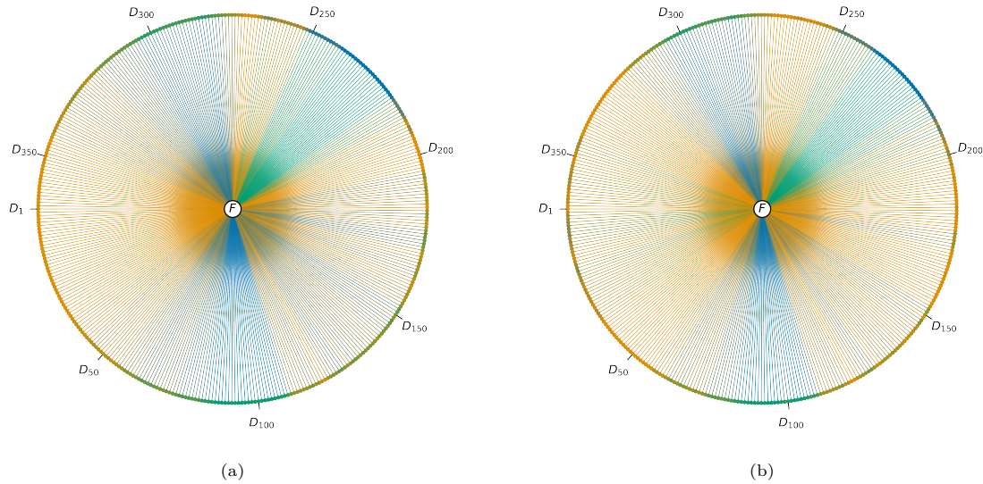
Figura 4: Aptitud diaria para la siembra en Brandeburgo, expresada como la probabilidad de transición \lambda_k , k \in \{1, 2, \dots, 365\} , calculada mediante las distancias Euclidiana y Manhattan. La figura 4a muestra los valores de \lambda_k calculados mediante la distancia Euclidiana, mientras que la figura 4b muestra los valores correspondientes calculados mediante la distancia Manhattan. La progresión del año se expresa en sentido contrario a las manecillas del reloj; en el exterior de la gráfica anular se indican los meses, mientras que en su interior se indican los días del año.
