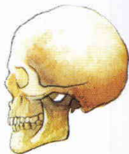
现代人
