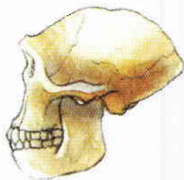
直立人
