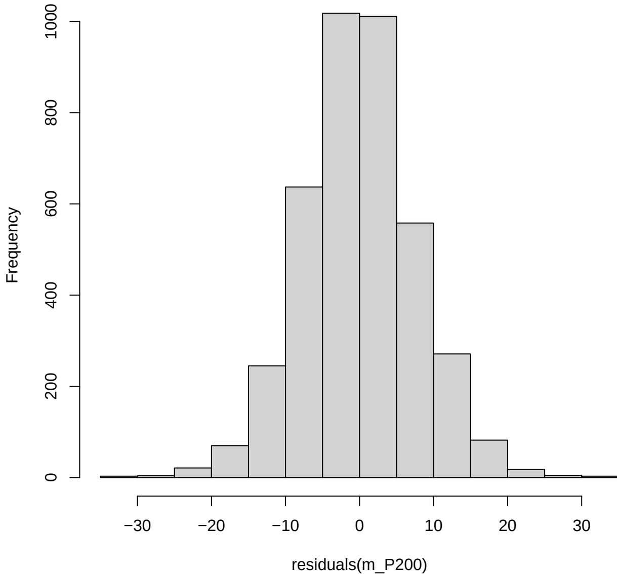
Histogram of residuals(m_P200)
