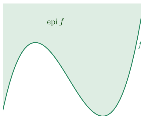
Figura 1.2.12: Epígrafo de una función f .
