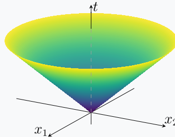
Figura 1.2.5: Cono de segundo orden \mathcal{Q}^3 asociado a la norma euclídea en \mathbb{R}^2 .
