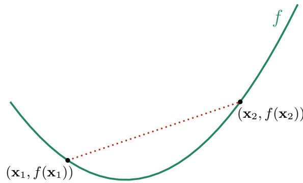
Figura 1.2.11: Grafo de una función convexa. La desigualdad (1.2.3) significa que el segmento de recta entre los puntos (\mathbf{x}_1, f(\mathbf{x}_1)) y (\mathbf{x}_2, f(\mathbf{x}_2)) se encuentra por encima de la gráfica de f .
