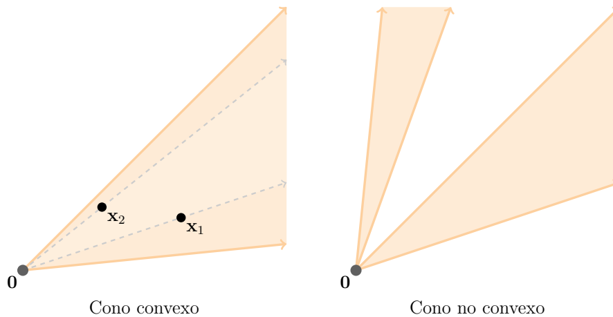
Figura 1.2.4: Ejemplo de un cono convexo y otro no convexo. En el caso de cono convexo, toda combinación lineal entre pares de puntos queda contenida en el cono.
