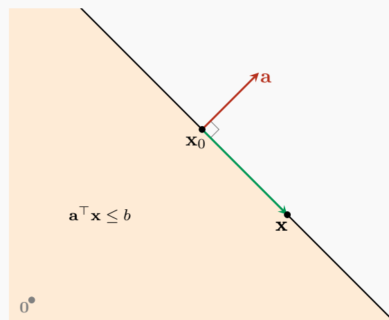
Figura 1.2.7: Hiperplano con vector normal \mathbf{a} .
