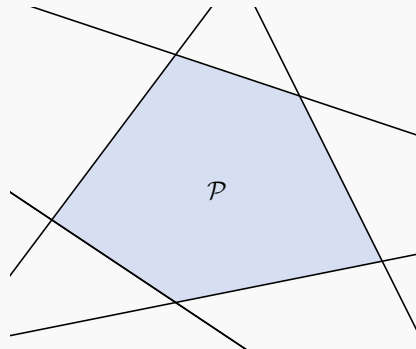
Figura 1.2.8: Un poliedro generado por la intersección de 5 semiespacios.
