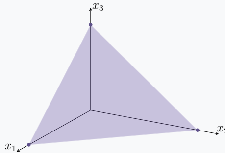
Figura 1.2.9: \Delta^2 es el triángulo en \mathbb{R}^3 de vértices (1, 0, 0) , (0, 1, 0) y (0, 0, 1) .
