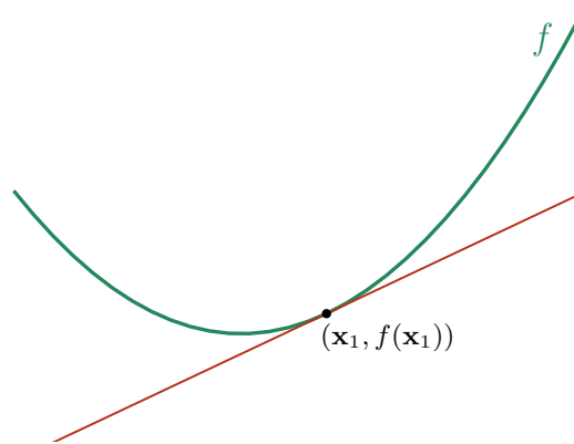
Figura 1.2.13: Grafo de una función convexa f y su aproximación lineal en \mathbf{x}_1 .
