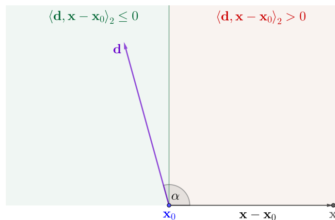
Figura 1.2.10: Interpretación geométrica de las direcciones \mathbf{d} y \mathbf{x} - \mathbf{x}_0 .
