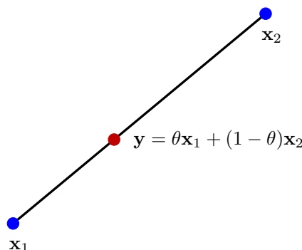
Figura 1.2.2: Combinación convexa entre dos puntos \mathbf{x}_1 y \mathbf{x}_2 .
