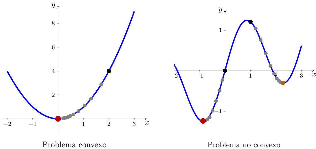
Figura 1.2.1: Comportamiento de un método iterativo en un problema de optimización.
