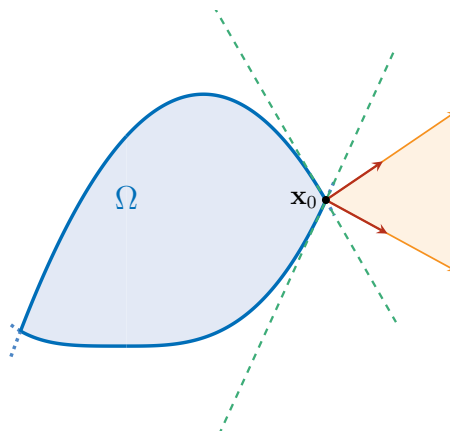
Figura 1.4.3: Cono normal de la linearización de restricciones activas en un punto \mathbf{x}_0 \in \Omega .
