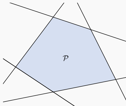
Figura 1.2.8: Un poliedro generado por la intersección de 5 semiespacios.
