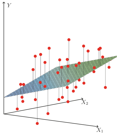
Figura 2.2.1: Interpretación geométrica del modelo de regresión lineal en \mathbb{R}^2 . El objetivo es hallar la función lineal de X que minimice la suma de los residuos al cuadrado respecto de Y . (Figura 3.1 de (Hastie, Tibshirani & Friedman 2009)).
