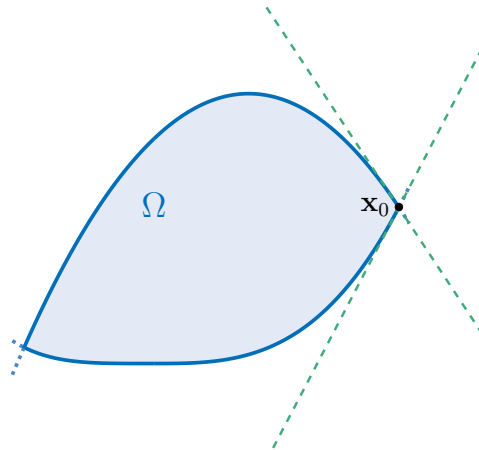
Figura 1.4.3: Linearización de restricciones activas en un punto \mathbf{x}_0 \in \Omega .
