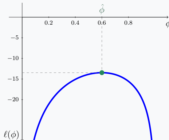
Figura 2.1.1: Función de verosimilitud para la distribución de Bernoulli con n = 20 y \sum_{i=1}^n y_i = 12 . El MLE resulta \hat{\phi} = 0.6 .
