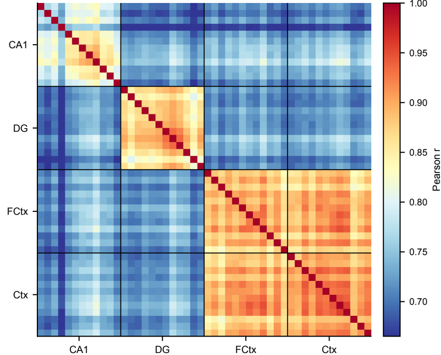
ROI × ROI correlation
