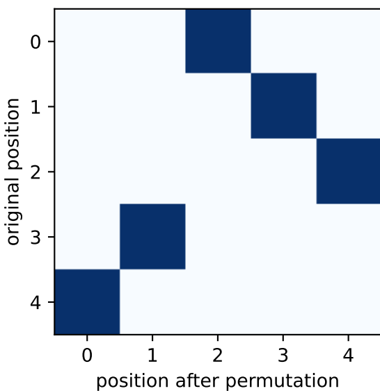
True \pi_S
