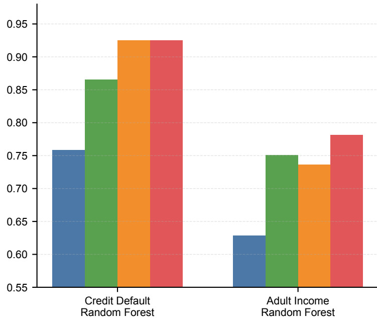
AUC
