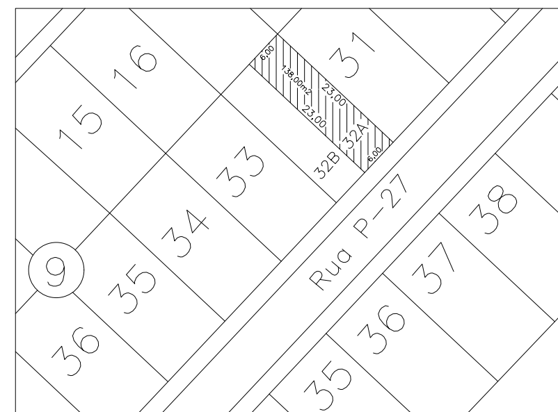
SITUAÇÃO – 1:75
