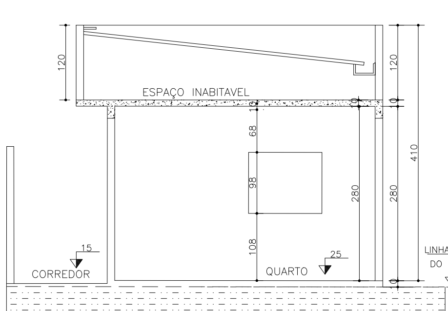
CORTE B B – 1:100
