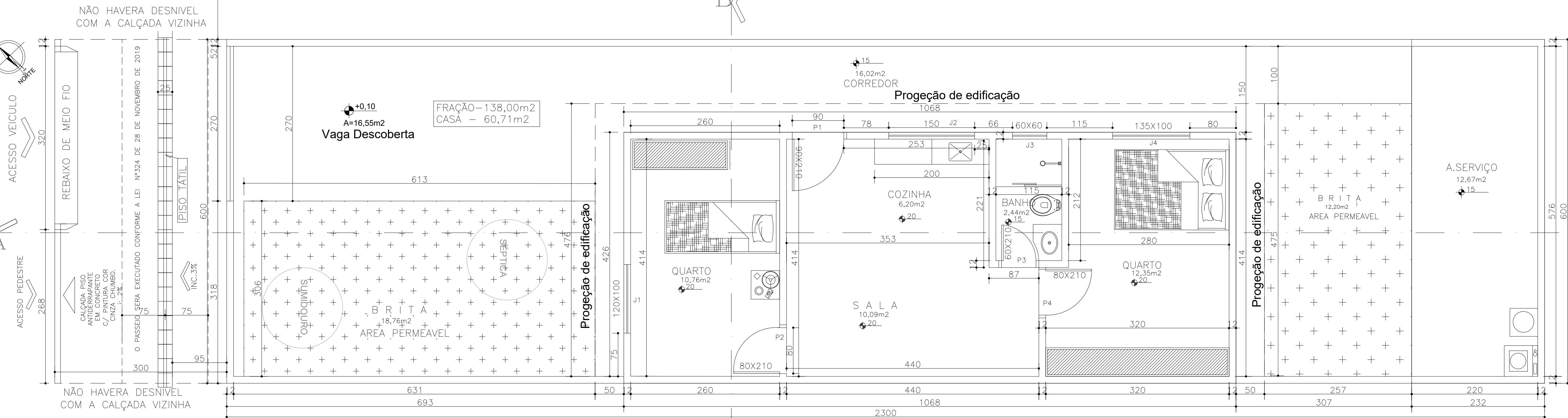
PLANTA BAIXA – 1:75
