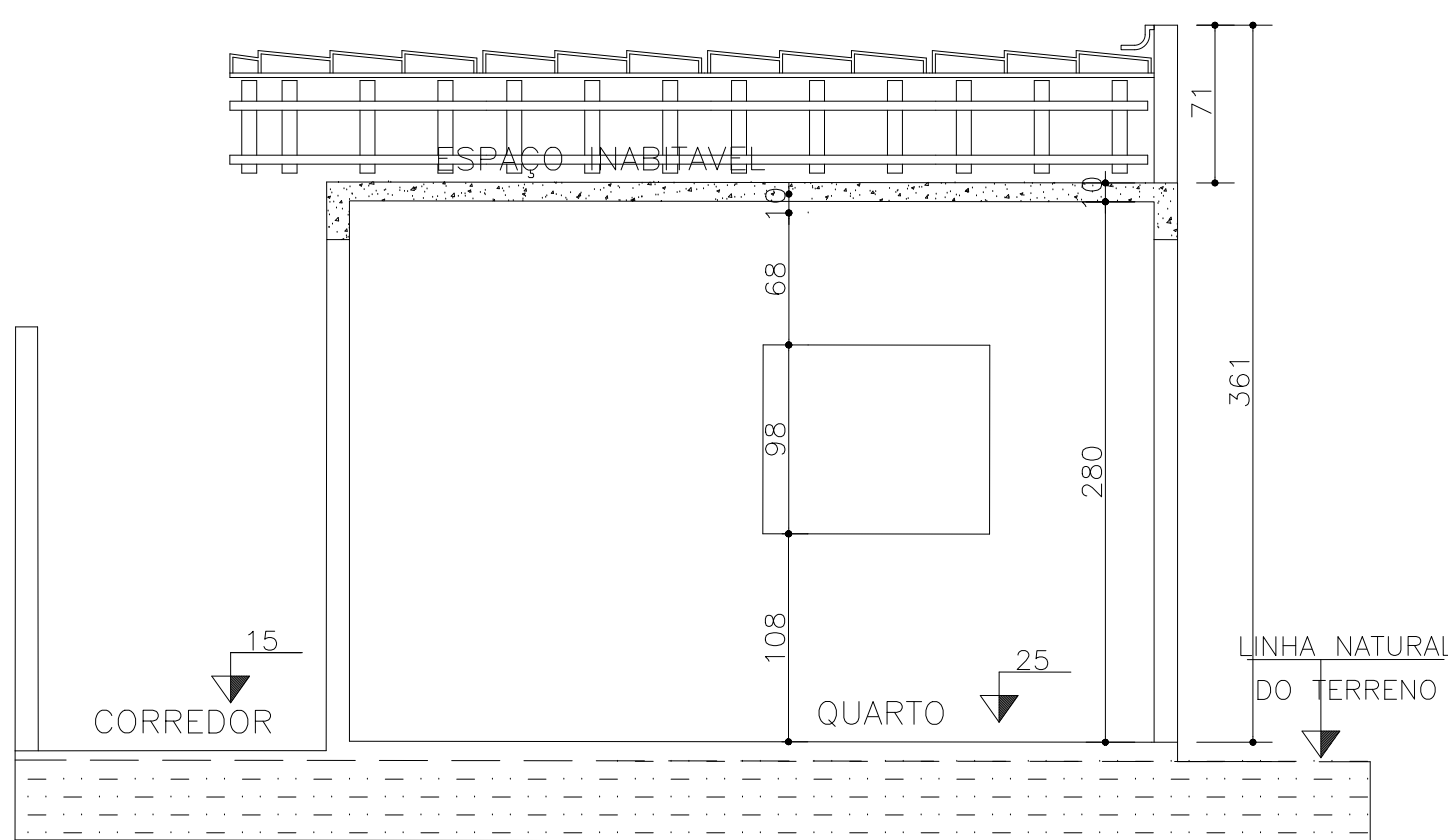
CORTE BB – 1:100
