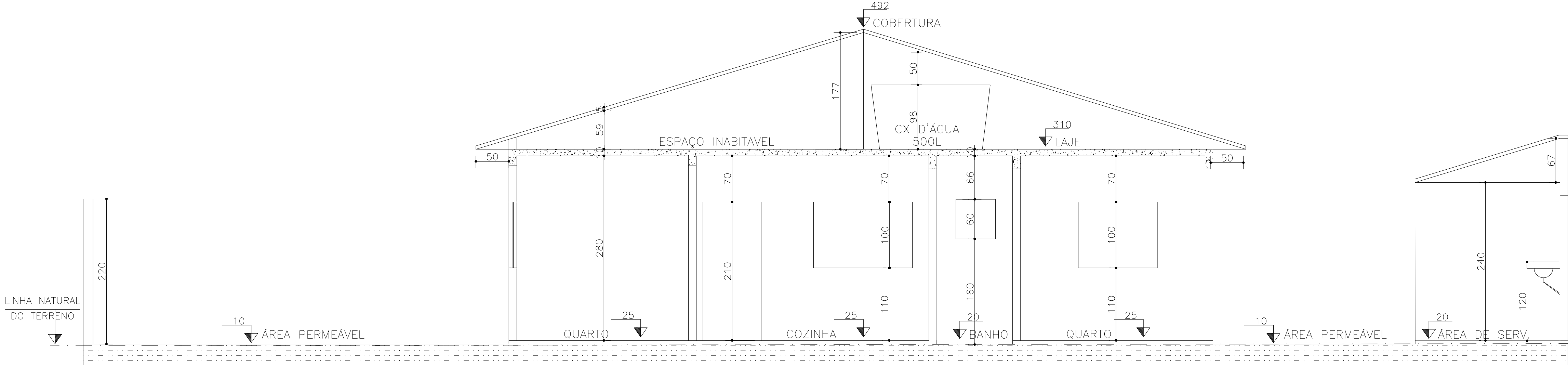
C O R T E A A – 1:100
