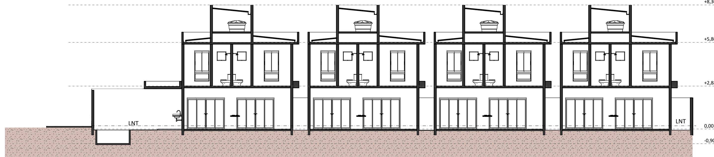
Corte AA- Locação
