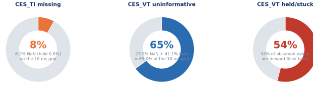
그림 1: 10 ms 격자에서의 CES 결측 구조. T_i 와 V_{rot} 은 독립적으로 결측되며 (8.2% / 23.9%), 행 필터링이 아닌 타겟별 마스킹을 요구한다. 계측기 유지값까지 세면 격자의 65.0% 가 독립적인 V_{rot} 정보를 갖지 않는다.
