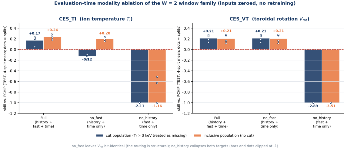
그림 5: 윈도 대조군의 평가 시점 모달리티 절제, 두 모집단. 고속 진단을 0 으로 만들면 V_{\text{rot}} 은 비트 단위로 동일하고 컷에서는 T_i 마진이 사라진다. 이력을 0 으로 만들면 두 타겟 모두 붕괴한다.
