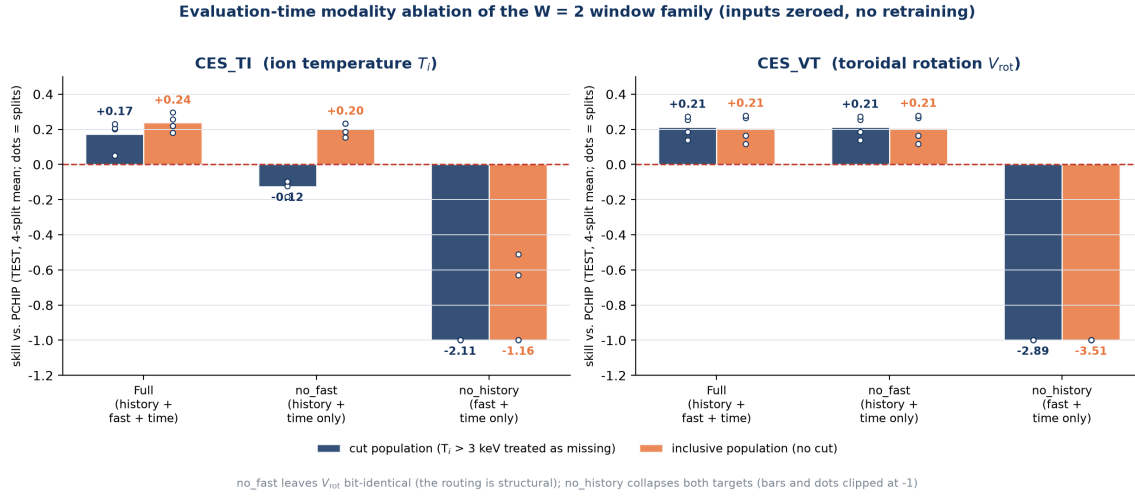
그림 5: 윈도우 대조군의 평가 시점 모달리티 절제, 두 모집단. 고속 진단을 0 으로 만들면 V_{\text{rot}} 은 비트 단위로 동일하고 컷에서는 T_i 마진이 사라진다. 이력을 0 으로 만들면 두 타겟 모두 붕괴한다.
