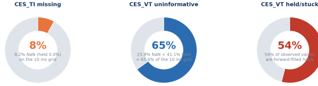
그림 1: 10 ms 격자에서의 CES 결측 구조. T_i 와 V_{\text{rot}} 은 독립적으로 결측되며 (8.2% / 23.9%), 행 필터링이 아닌 타겟별 마스킹을 요구한다. 계측기 유지값까지 세면 격자의 65.0% 가 독립적인 V_{\text{rot}} 정보를 갖지 않는다.
