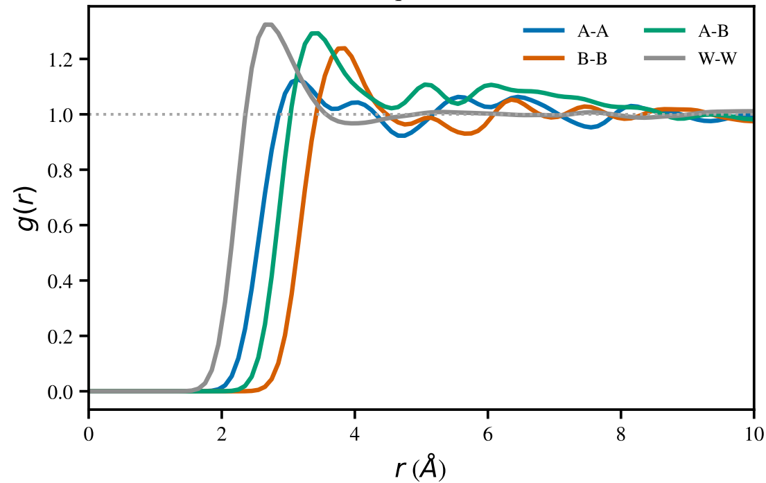
All-atom equilibrium RDFs
