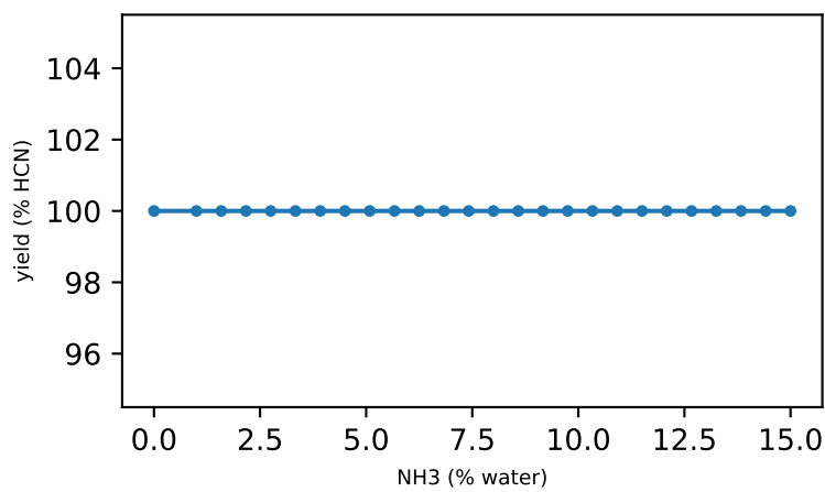
asparticacid
