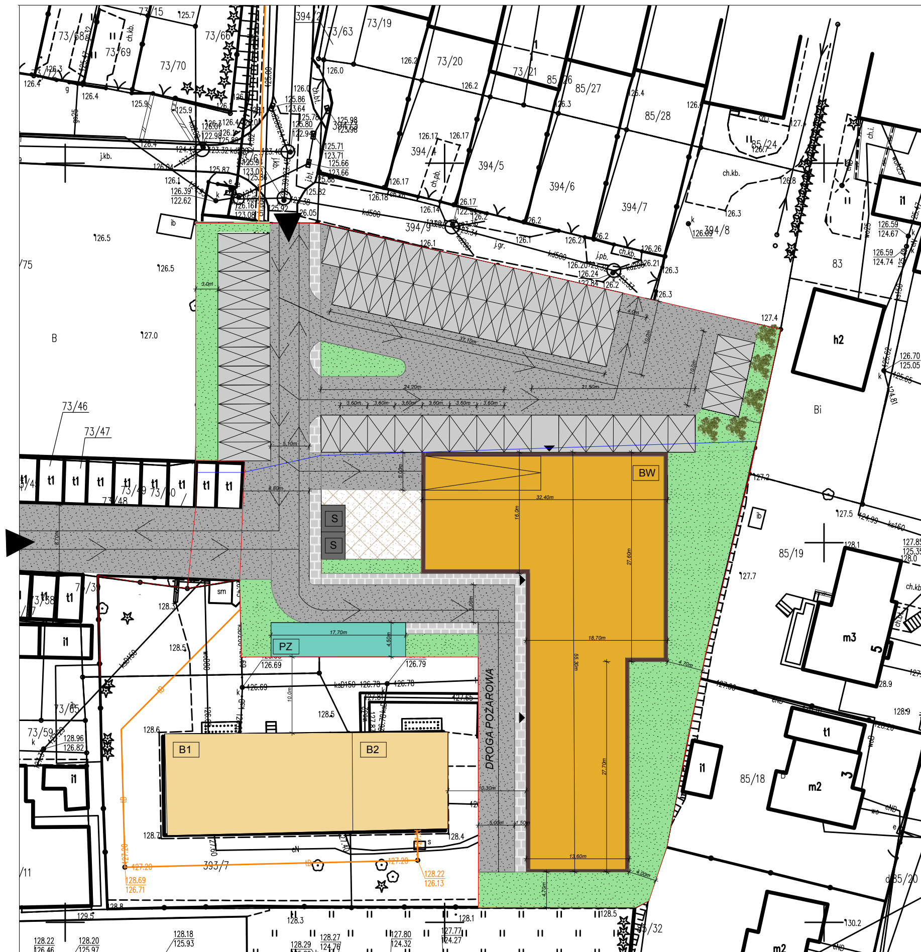
KONCEPCJA ZAGOSPODAROWANIA BARCZEWO dz.nr 393/1, obr.2, m. Barczewo.
