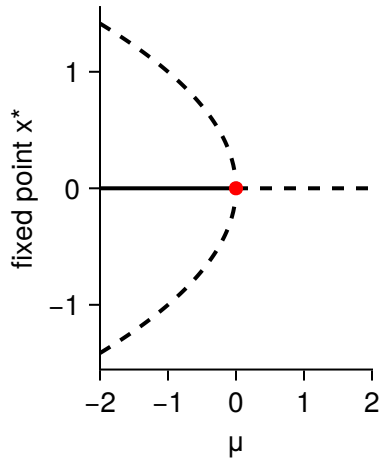
(d) subcritical pitchfork
