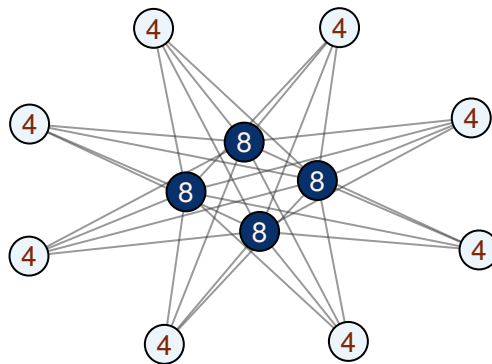
(b) complete bipartite (N=12)
