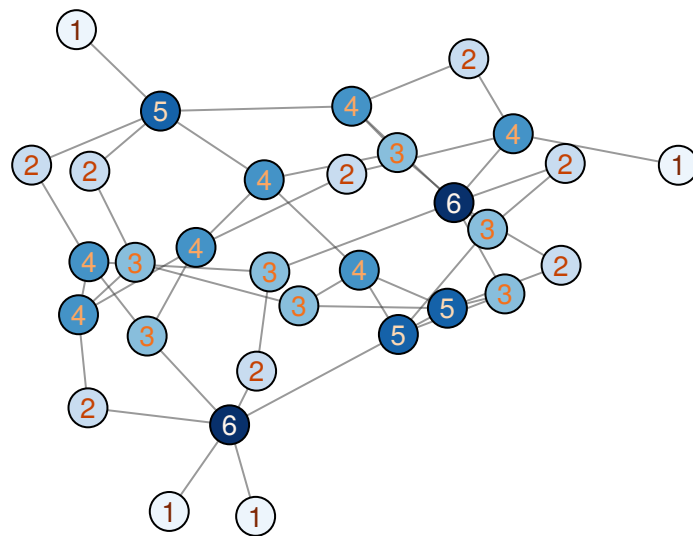
(e) Erdős-Rényi (N=31)
