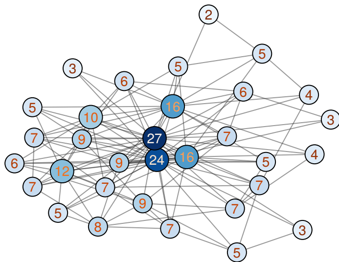
(d) static scale-free (N=32)
