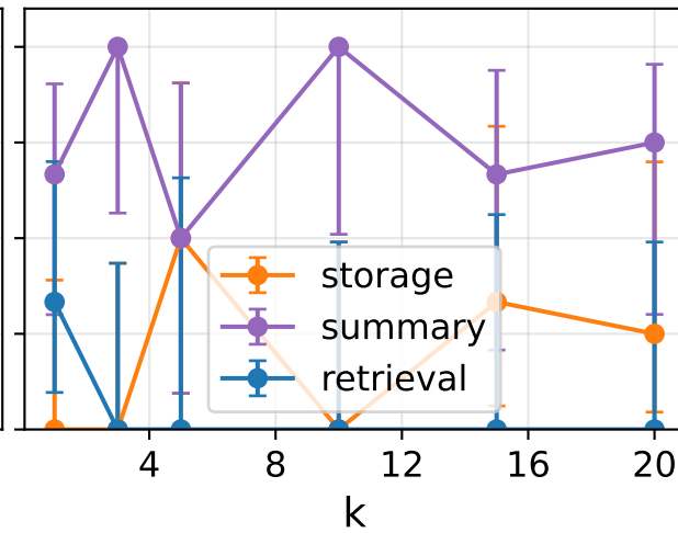
A-MEM
