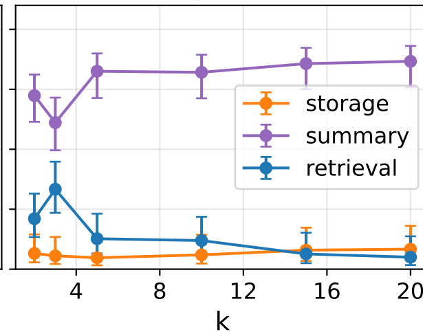
SimpleMem
