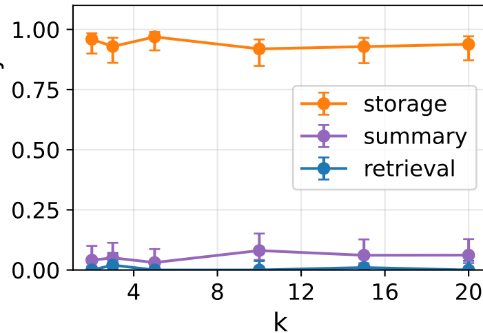
Mem0
