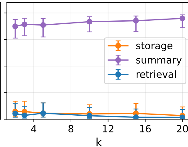
A-MEM
