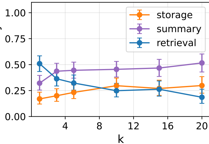
Mem0
