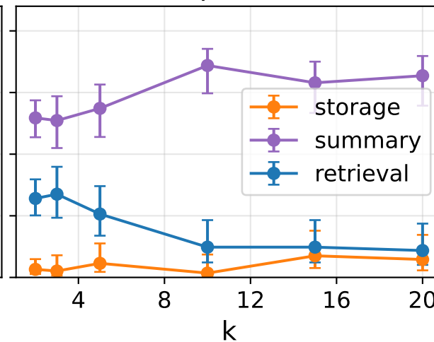
SimpleMem
