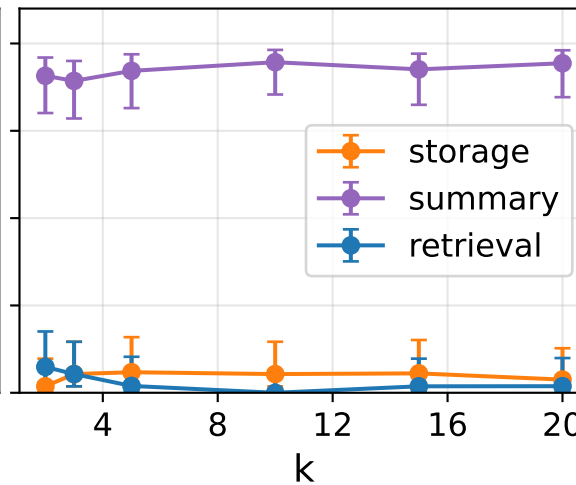
A-MEM
