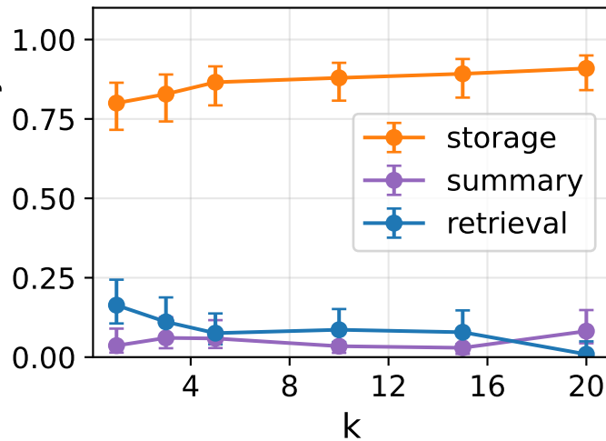
Mem0
