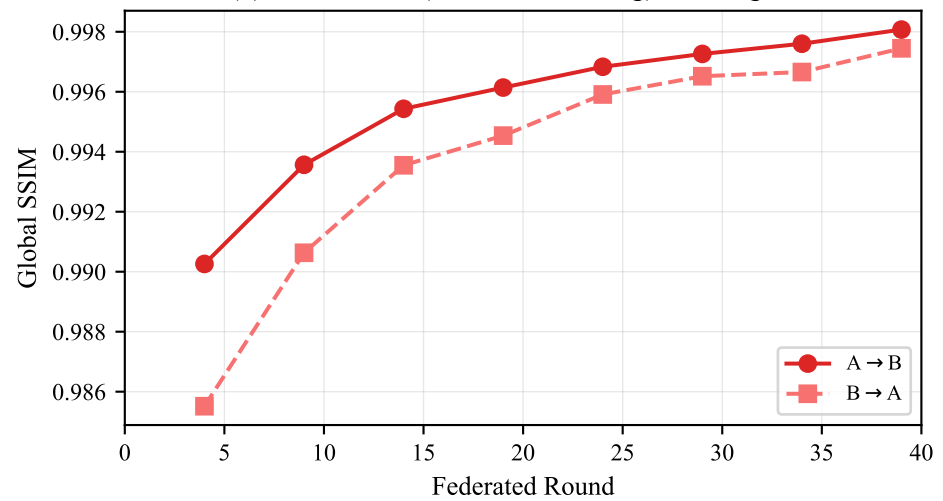
(d) Extension E (Federated FedAvg) Convergence
