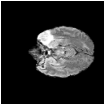
raw FLAIR
