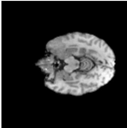
raw T1
