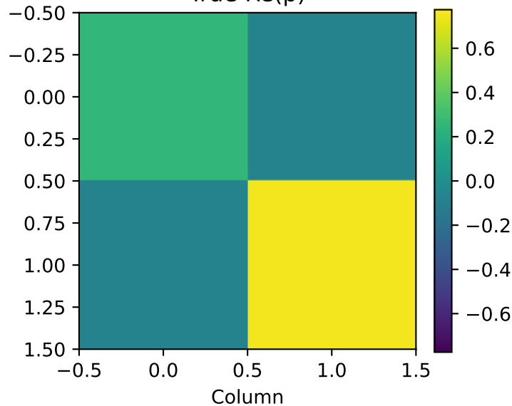
True \text{Re}(\rho)
