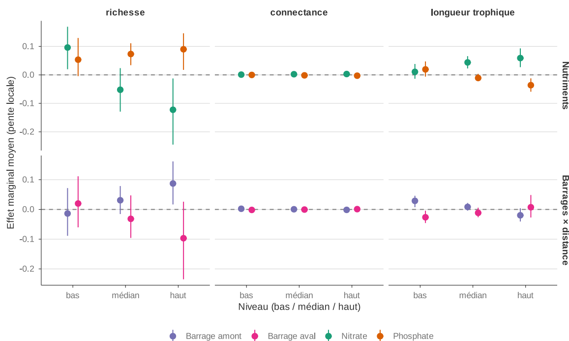
Figure 7. Effet marginal moyen (AME) du nitrate et du phosphate (auto-interaction, ligne du haut) et des deux effets barrage (interaction avec la distance à l'embouchure, ligne du bas), sur les trois métriques de structure des réseaux trophiques (colonnes). Barres verticales : intervalle de crédibilité à 95%.
